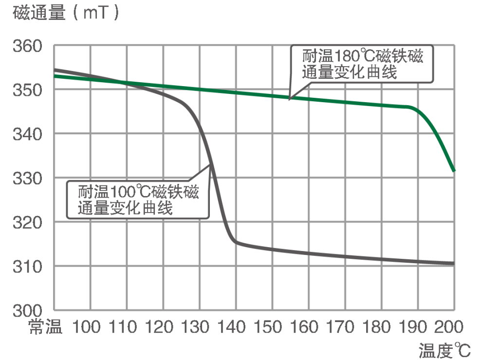
Magnetic flux comparison chart 磁铁磁通量耐温变化对比曲线
